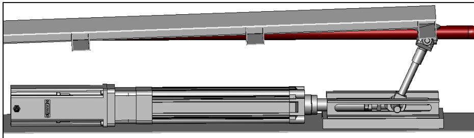
Figure 11 : Vérin placé sous le plateau et renvoi d'angle
