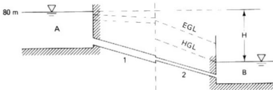
Figure 1 : Une conduite, deux réservoirs
